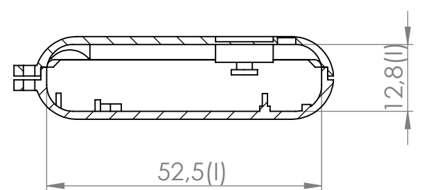
Sección/Section Q-Q
