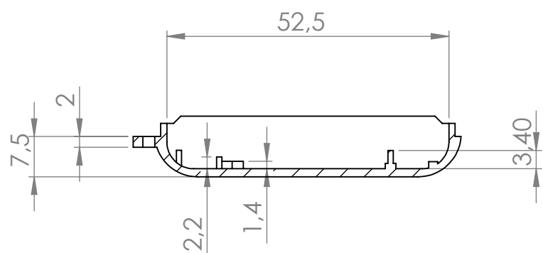
Sección/Section S-S
